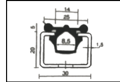
Schalldämmungs-Einlegegummi RU 25
