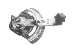
Klappensteller KV
