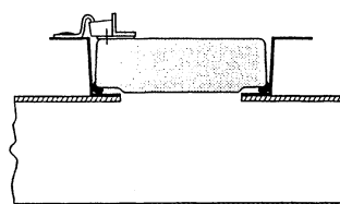
Montage à l'extérieur de la gaine (gainnes non isolées)
