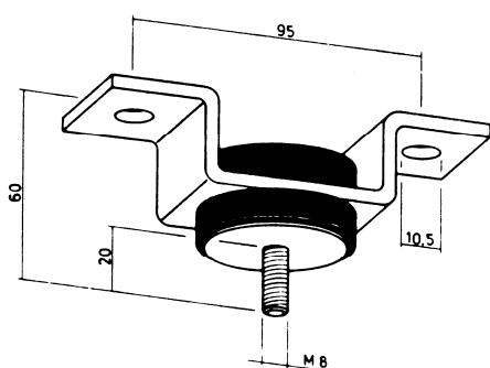
Réf. 652/M8 avec vis M8 x 45 Réf. 652/M10 avec vis M10 x 45 Elément insonorisant avec filetage extérieur, charge pour traction et pression de 75-150 kg (750-1500 N) Promatisé
