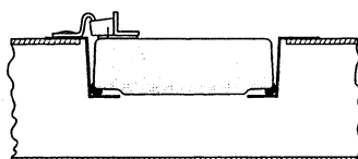
Montage à l'intérieur de la gaine (gainnes non isolées)
